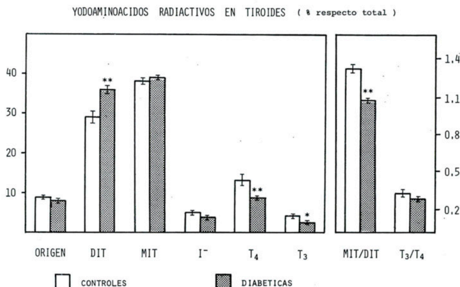
FIG. 1.— Distribución porcentual de los yodoaminoácidos radiactivos en el tiroides a las 24 horas de la inyección i.p. de yoduro- I^{131} en ratas que habían sido tratadas con una dosis única de estreptozotocina (70 mg/kg de peso corporal) y en controles. Media \pm E.S.M. de 4-14 ratas/grupo. Los asteriscos corresponden a la diferencia estadística entre ambos grupos: * = p < 0,05 , ** = p < 0,01 .
